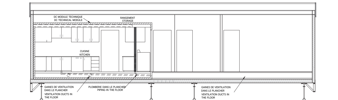
COUPE BB' SECTION BB'
