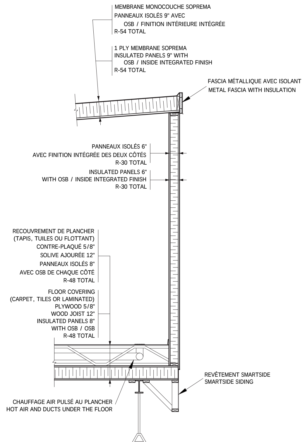
COUPE OPTIONS 3-4 SECTION OPTIONS 3-4
