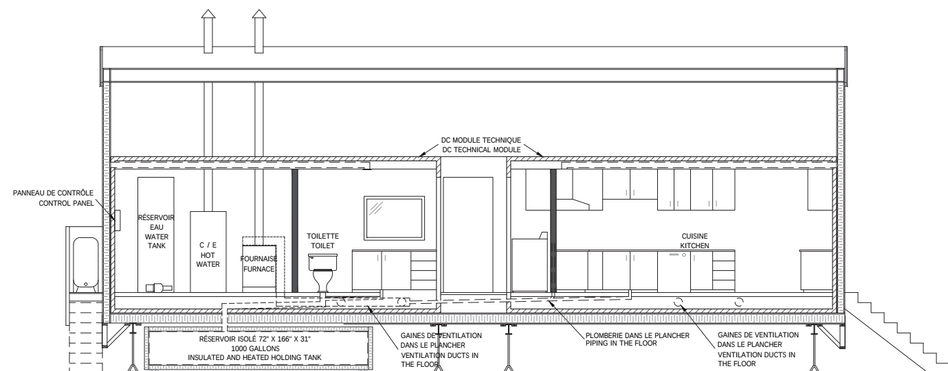
COUPE BB' SECTION BB'
