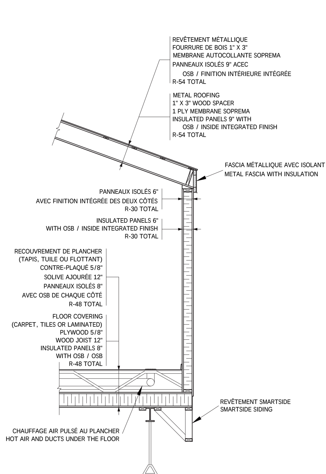
COUPE OPTIONS 1-2 SECTION OPTIONS 1-2
