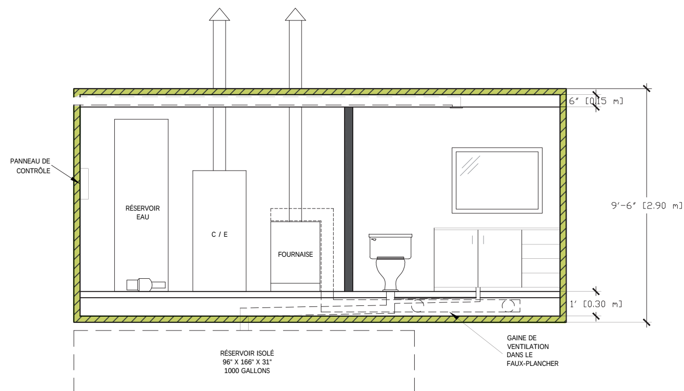
COUPE MODULE 1 - SALLE MÉCANIQUE SECTION MODULE 1 - MECHANICAL ROOM
