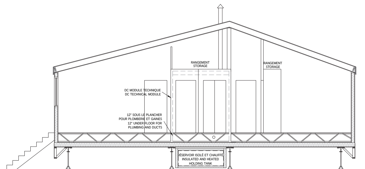
COUPE AA' SECTION AA'
