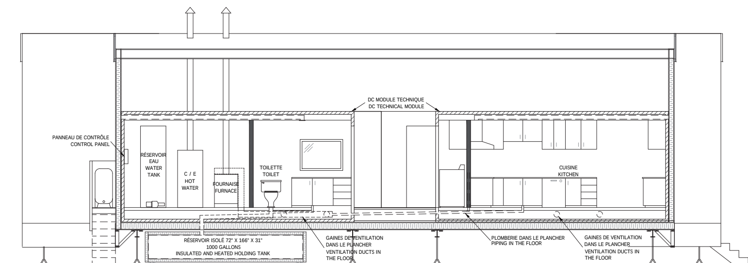
COUPE BB' SECTION BB'
