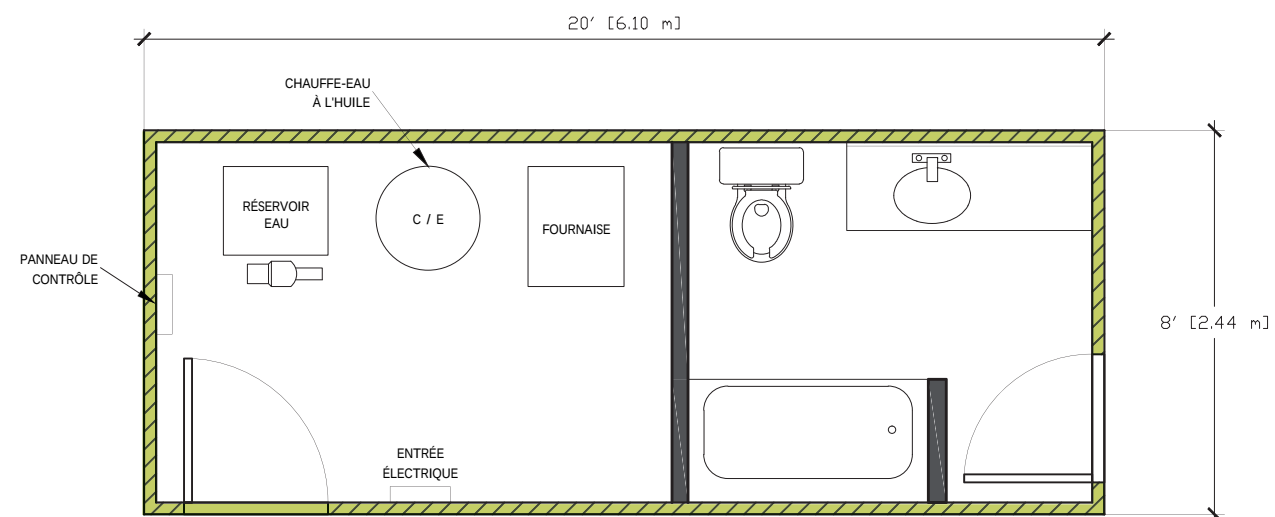
PLAN MODULE 1 - SALLE MÉCANIQUE PLAN MODULE 1 - MECHANICAL ROOM
