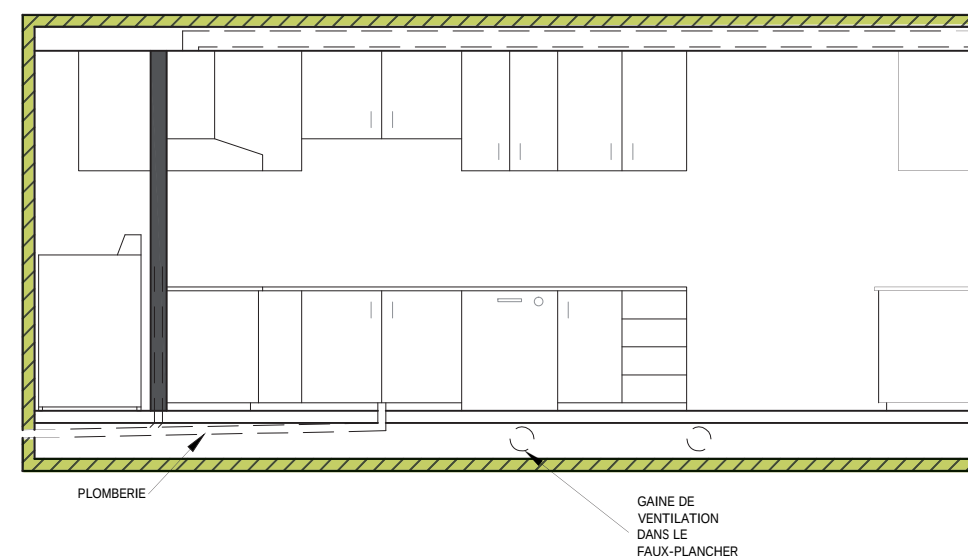
COUPE MODULE 1 - CUISINE SECTION MODULE 1 - KITCHEN
